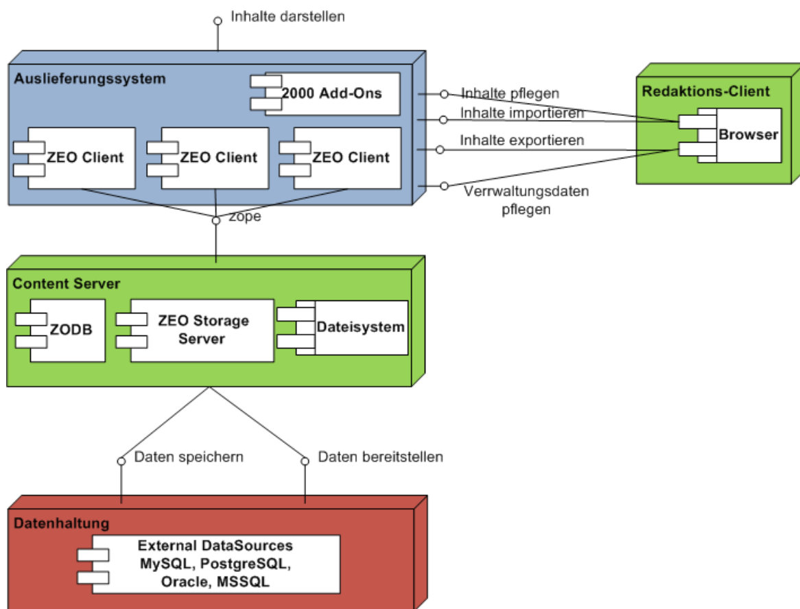
Abbildung 2.3: Plone – Systemarchitektur
